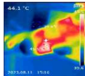
อุณหภูมิสายดิน INVERTER 45.5 °C 18SNPB-WIV01
