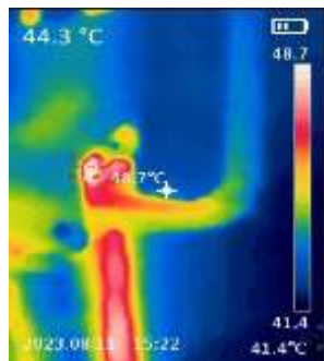
ตรวจสอบความร้อนสายฟิวส์ MCCB 48.7 °C
